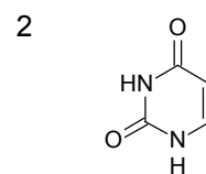
Uracil
