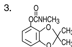
Bendiocarb
