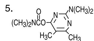
Pirimicarb
