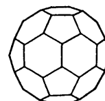
Buckminsterfullerene(C60)
